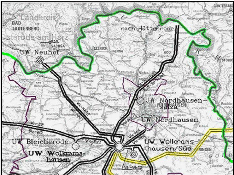
Bild 7: 110-kV-Doppelleitung Wolkramshausen–Neuhof
